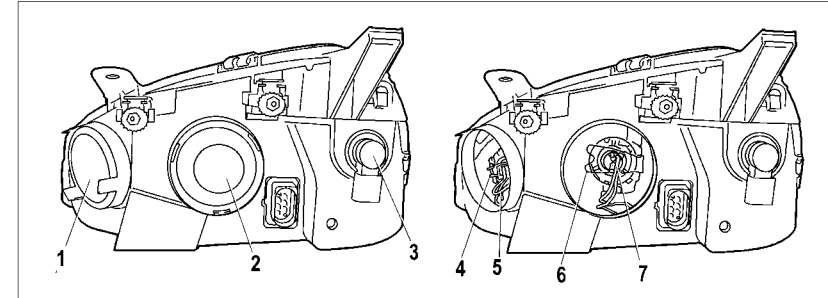
Рис. 51. Блок-фара
