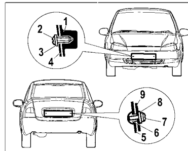
Рис. 38. Крепление номерных знаков
