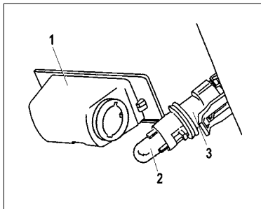
Рис. 54. Фонарь освещения номерного знака
