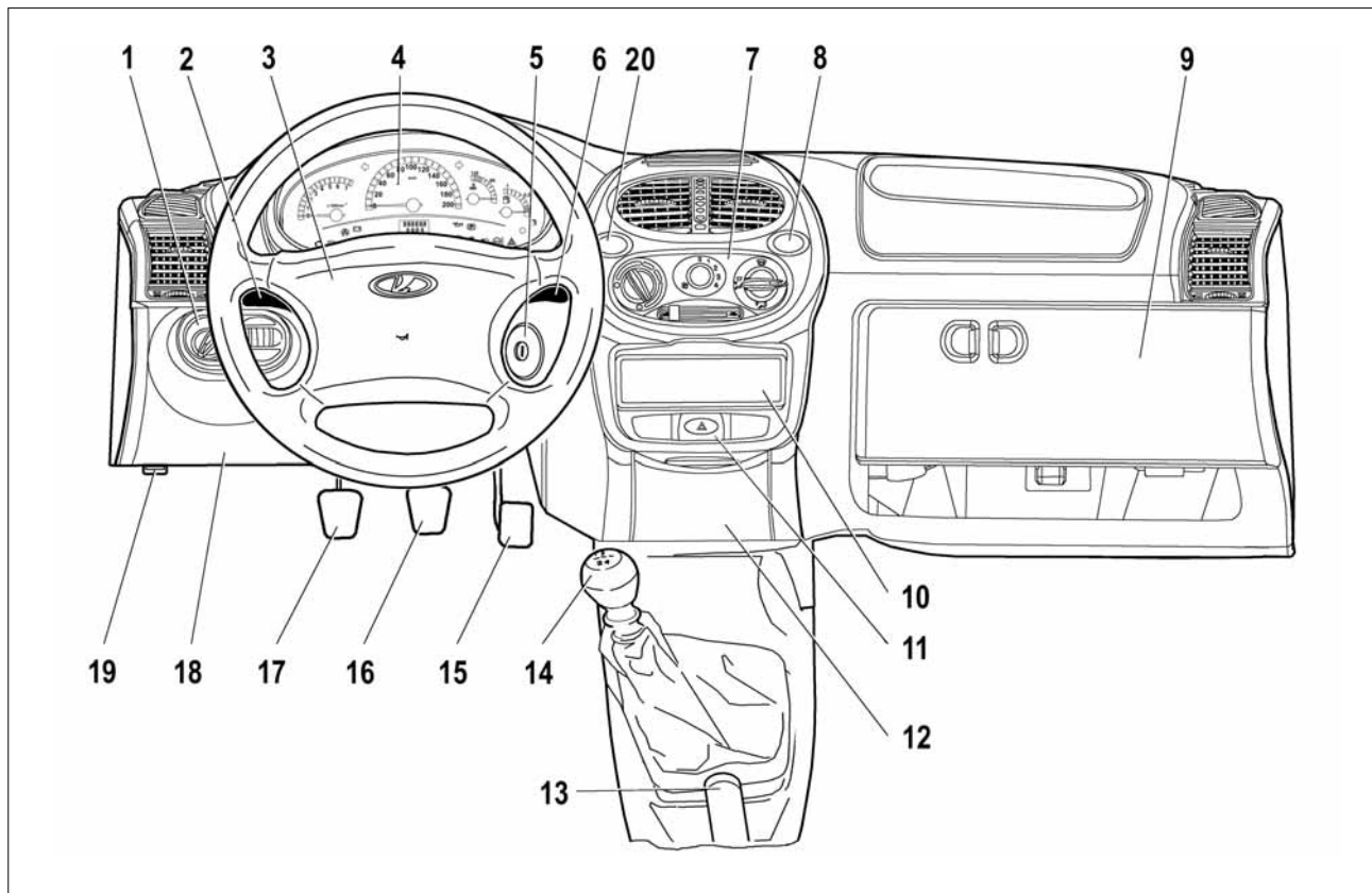
Рис. 28. Панель приборов
