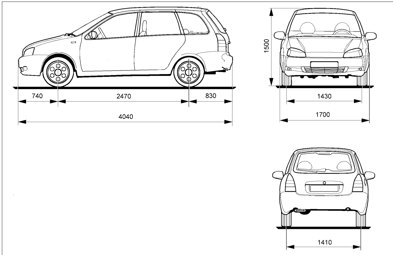
Рис. 58а. Габаритные (справочные) размеры автомобиля ВАЗ-11173 и его модификаций
