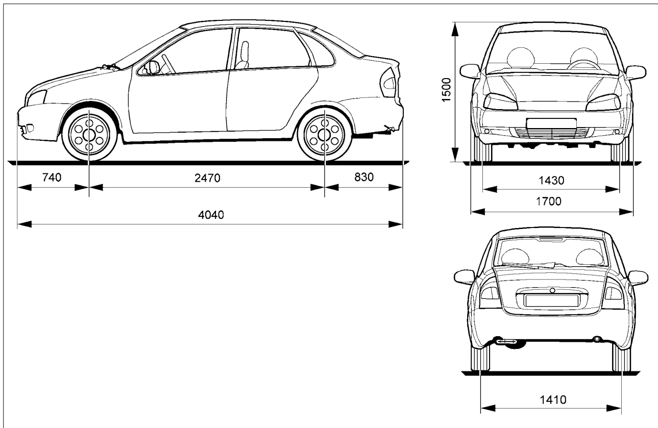
Рис. 586. Габаритные (справочные) размеры автомобиля ВАЗ-11183 и его модификаций
