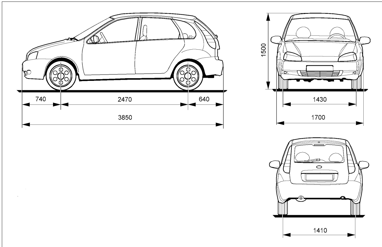
Рис. 58в. Габаритные (справочные) размеры автомобиля ВАЗ-11193 и его модификаций
