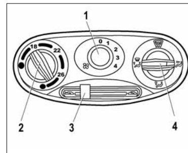
Рис. 36б. Блок управления системой вентиляции и отопления (в варианном исполнении)
