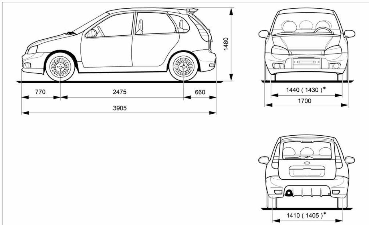
Рис. 58г. Габаритные (справочные) размеры автомобиля LADA KALINA Sport
