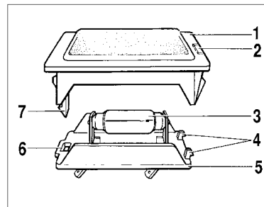
Рис. 56. Фонарь освещения вещевого ящика
