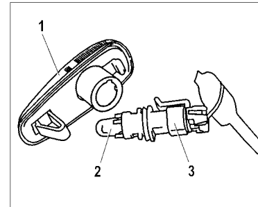
Рис. 53. Боковой указатель поворота
