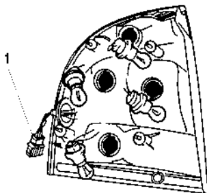
Рис. 52. Задний фонарь
