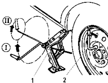
Рис. 47. Подъем автомобиля при замене колес
