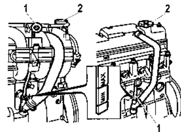
Рис. 40. Проверка уровня масла в картере двигателя
