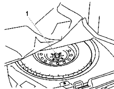
Рис. 48. Укладка запасного колеса
