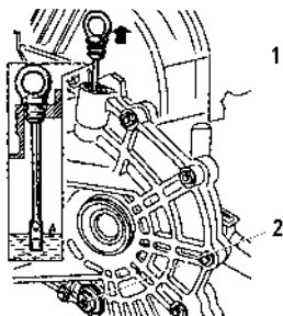
Рис. 41. Проверка уровня масла в коробке передач
