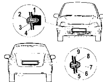
Рис. 38. Крепление номерных знаков
