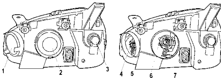
Рис. 51. Блок-фара
