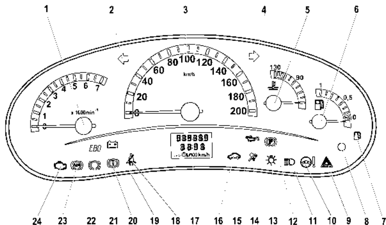
Рис. 29. Комбинация приборов
