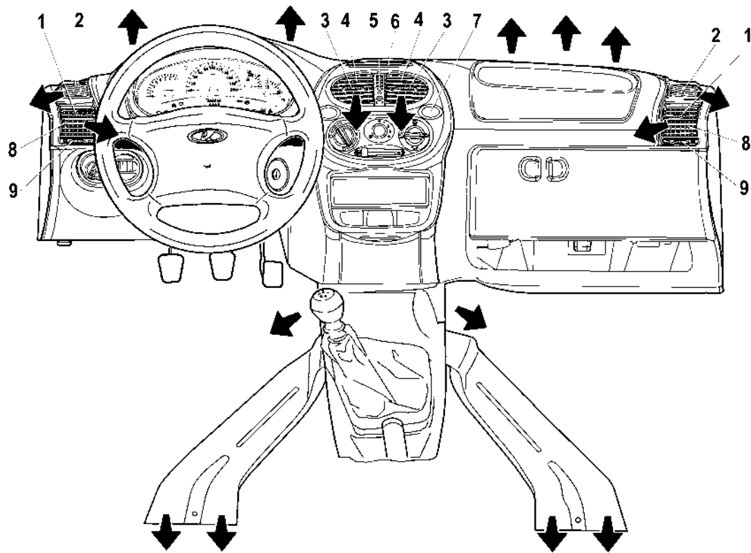
Рис. 37. Органы управления вентиляцией
